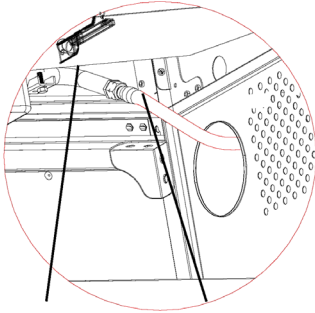
Conector de gas Manguera
